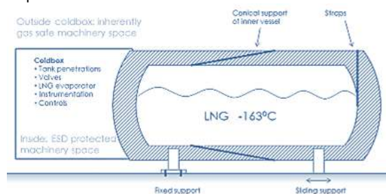
Figure 2.27 – LNG Type-C Tank
